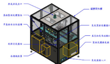
大氣式原子層沉積設備
