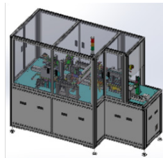
微投影機鏡片組裝設備
