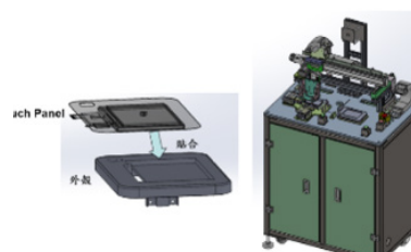
觸控面板組裝設備
